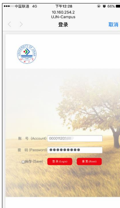
图 1-2 登录界面
